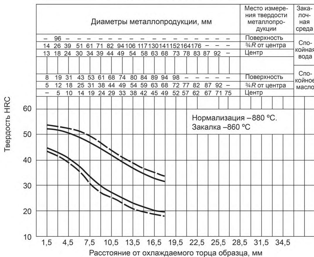
Рисунок А.4 — Сталь марки 35Х
