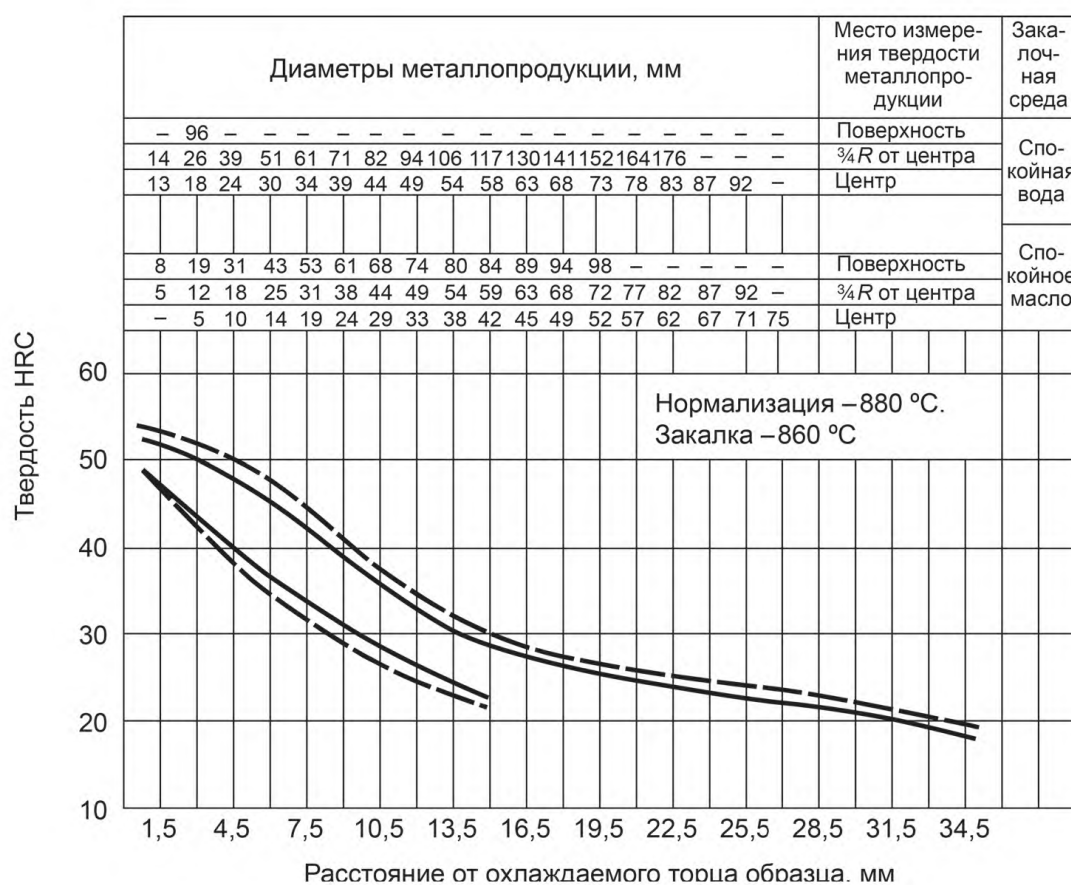
Рисунок А.3 — Сталь марки 30Х
